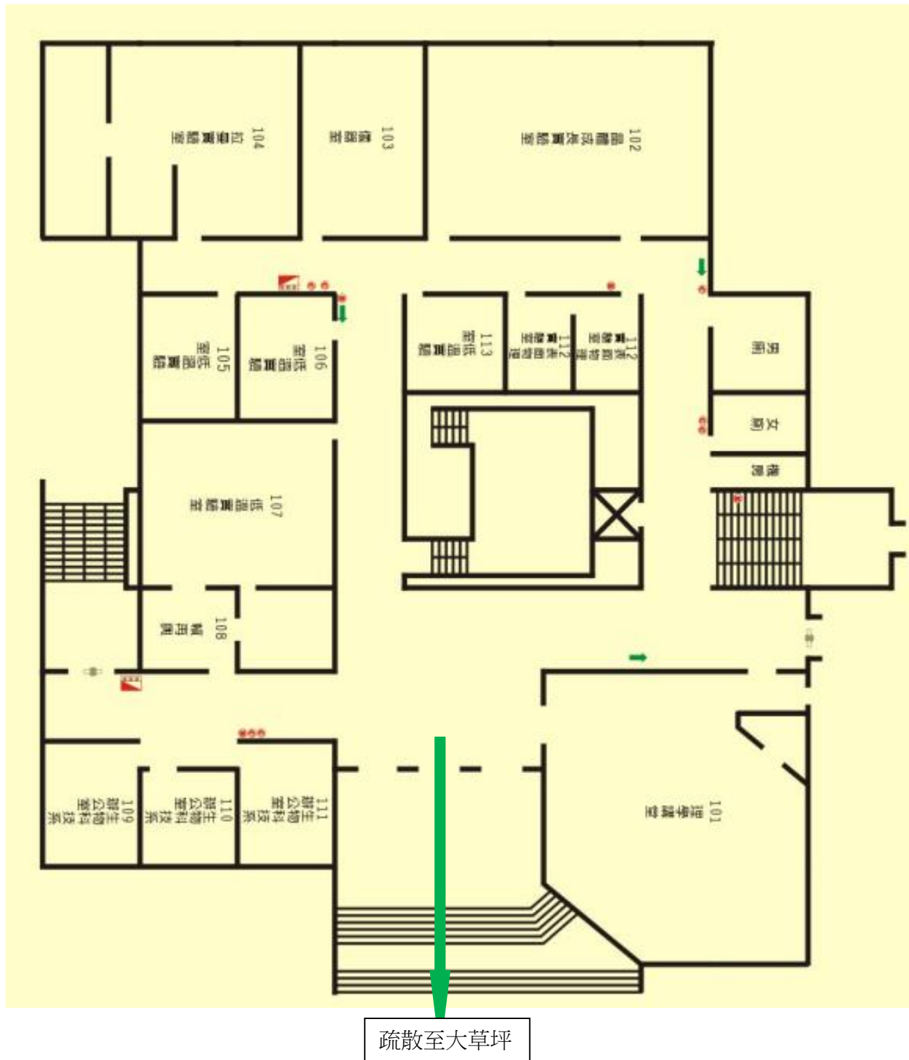
理學館 1 樓消防設備平面圖
